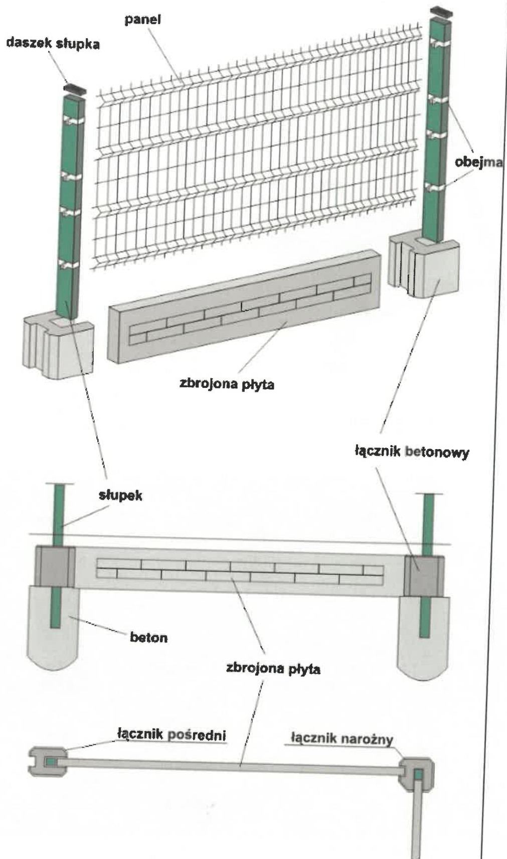
Rys. 3. Rysunek poglądowy ogrodzenia panelowego
